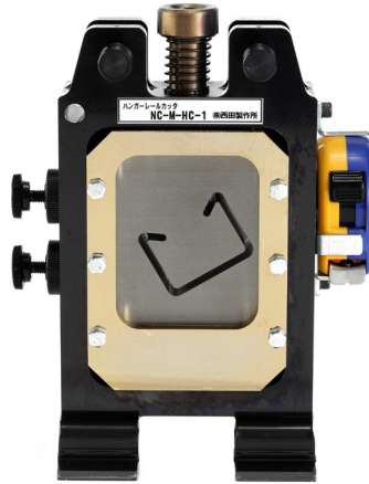
本体フレームに切断刃物がセットされた状態
